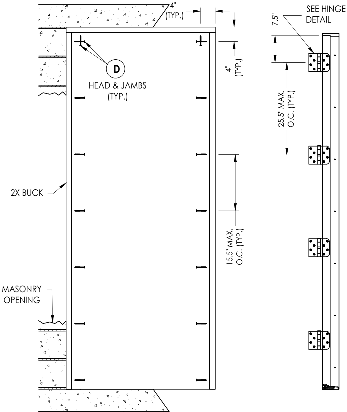
HINGE JAMB
